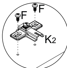
Detalhe 6 Detail/Detalle
